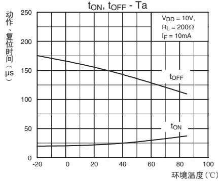
动作、复位时间—环境温度
